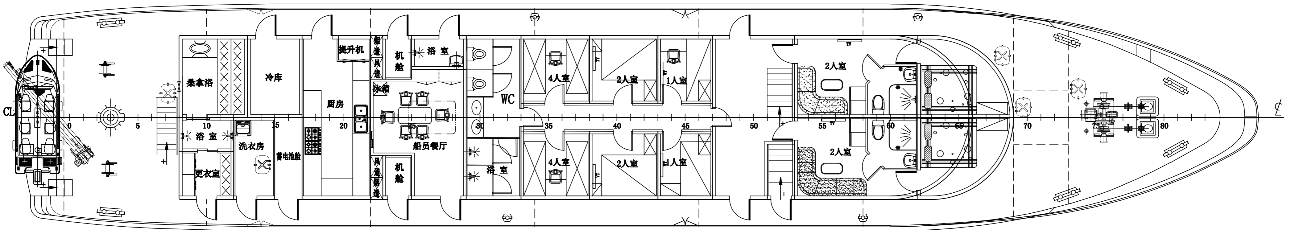
底舱
