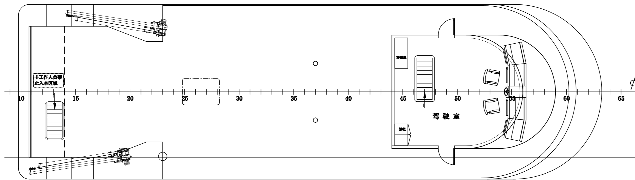
驾驶甲板
