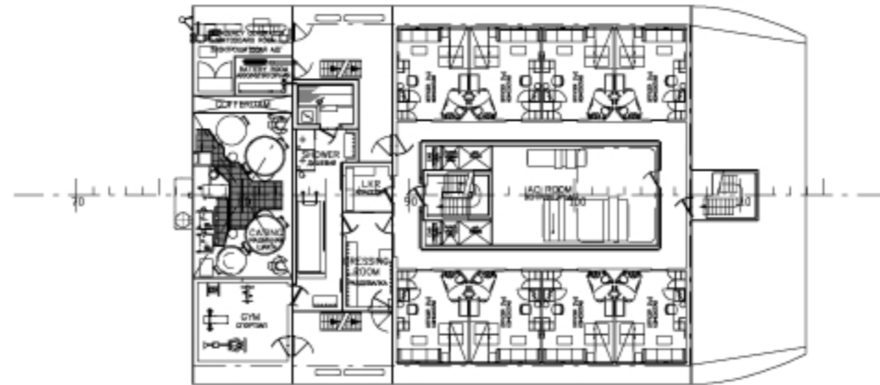
2ND BRIDGE DECK (Deck 7) 109,10 м² 2-Я ПАЛУБА НАДСТРОЙКИ (ПАЛУБА 7)
