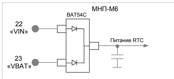
Рисунок 2 — Питание RTC в МНП-М6
