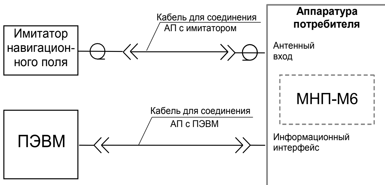
Рисунок 10 – Схема подключения МНП-М6 при работе с имитатором навигационного поля
