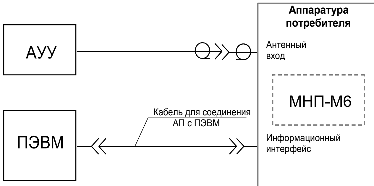
Рисунок 9 – Схема подключения МНП-М6 при работе по реальному сигналу
