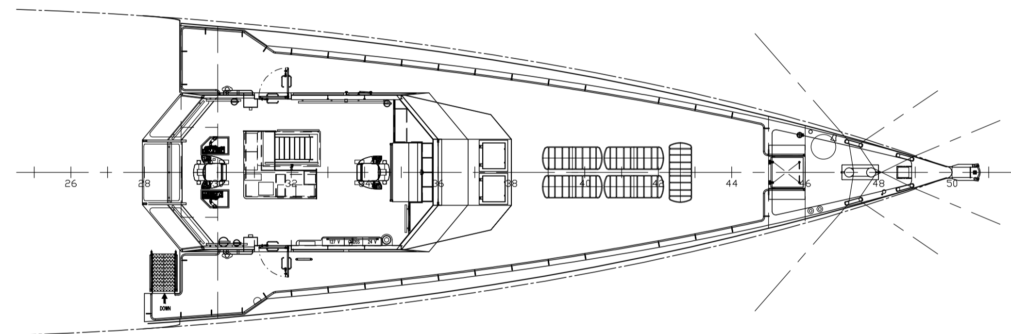
Bridgedeck
