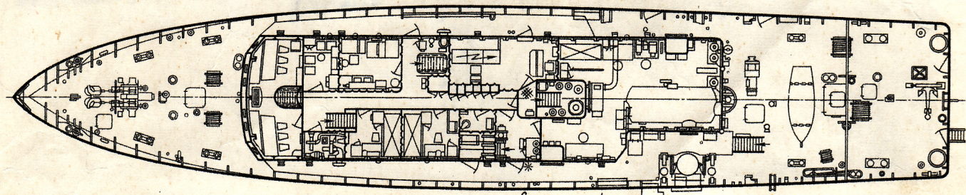
Верхняя палуба
