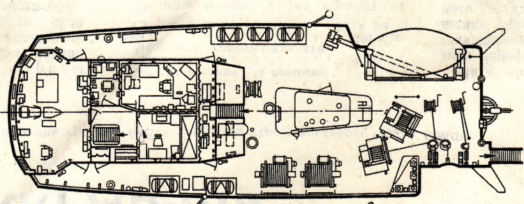
Палуба надстройки
