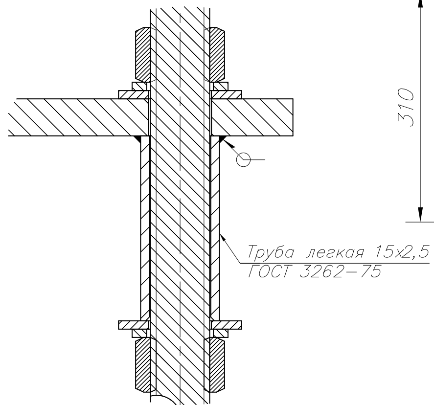
Узел А (1:1)
