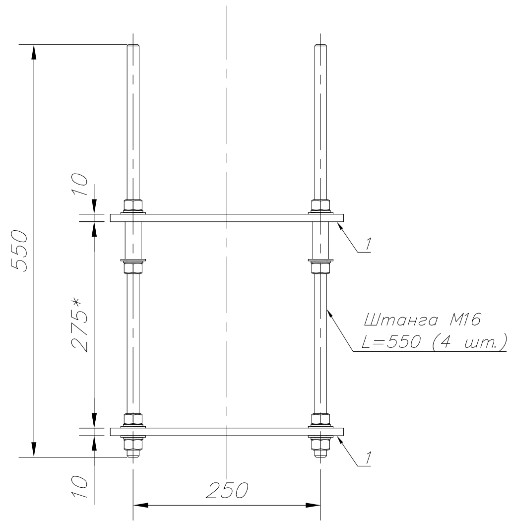
Узел А (1:1)
